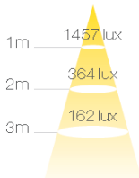
ILLUMINANCE(lux)
